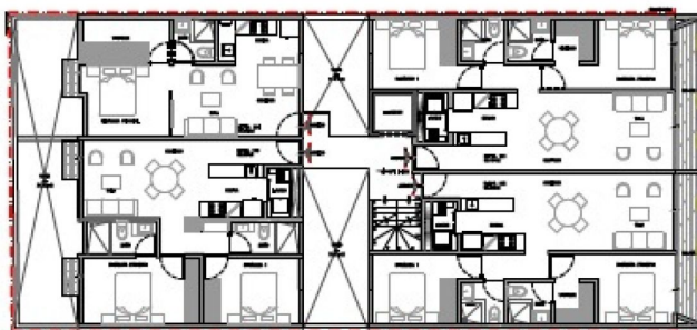
PLANTA TIPO
